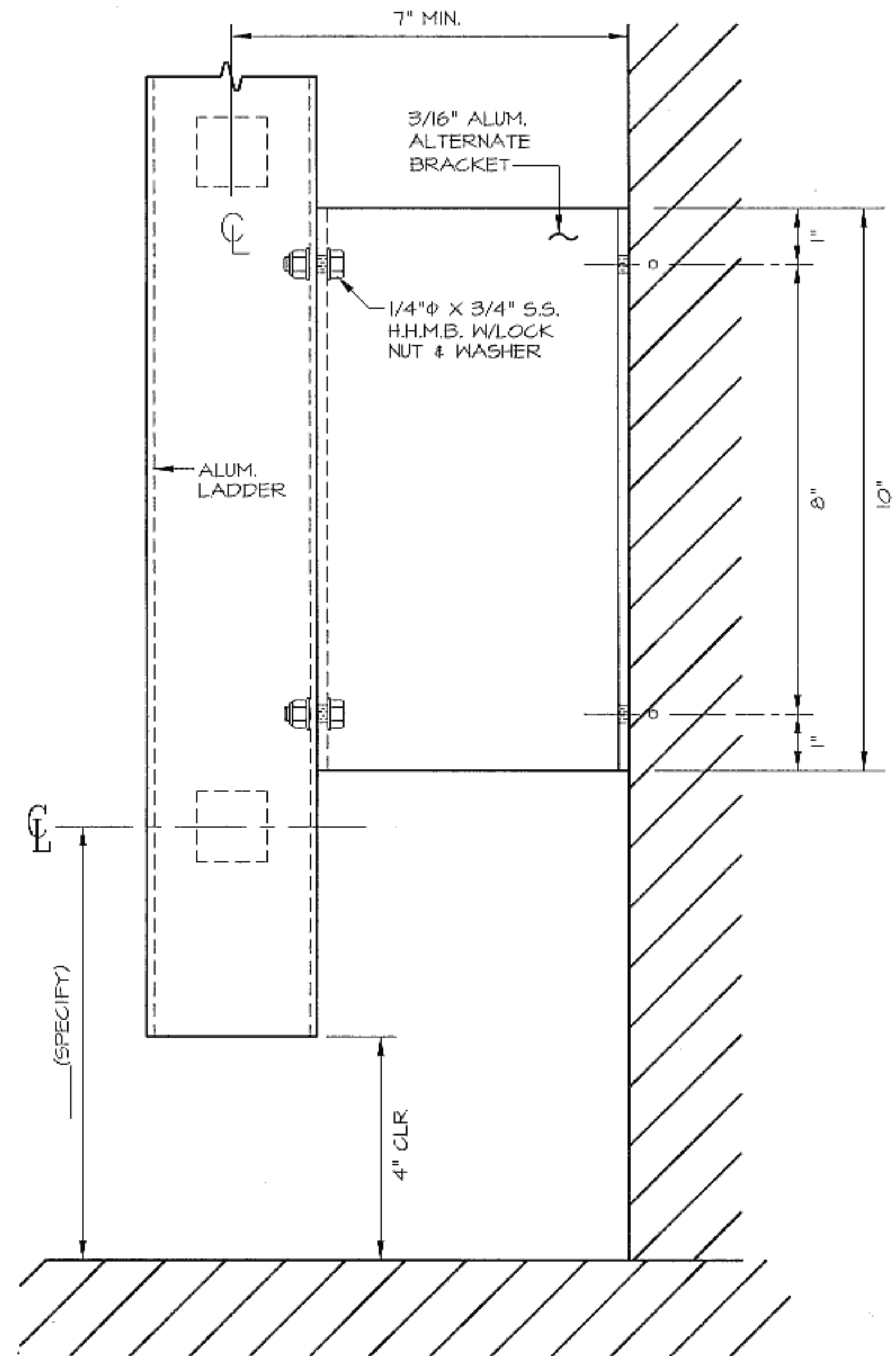
ALTERNATE BOTTOM BRACKET SCALE: 3"=1'-0"
