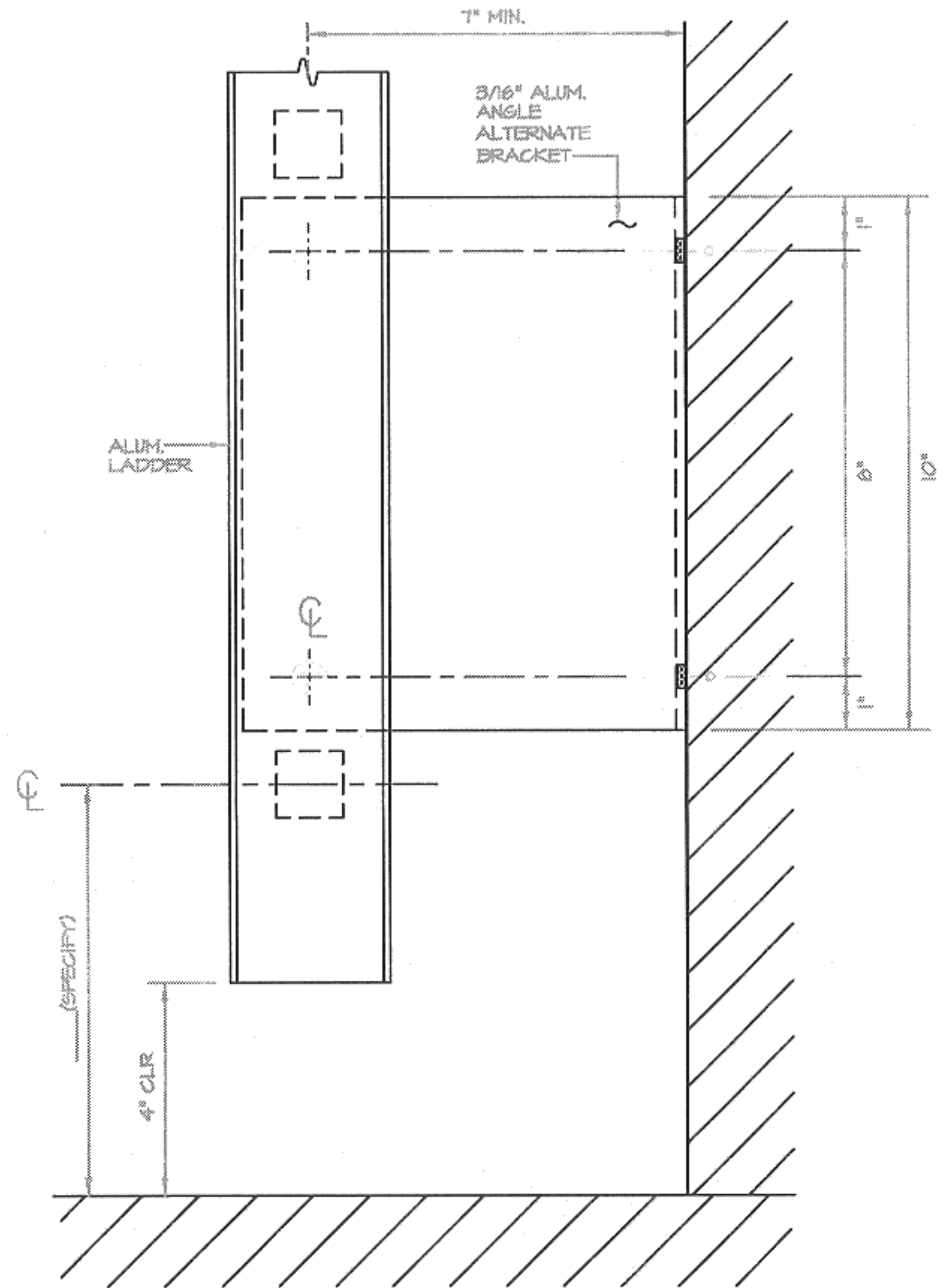
ALTERNATE BOTTOM BRACKET SCALE: 3"=1'-0"
