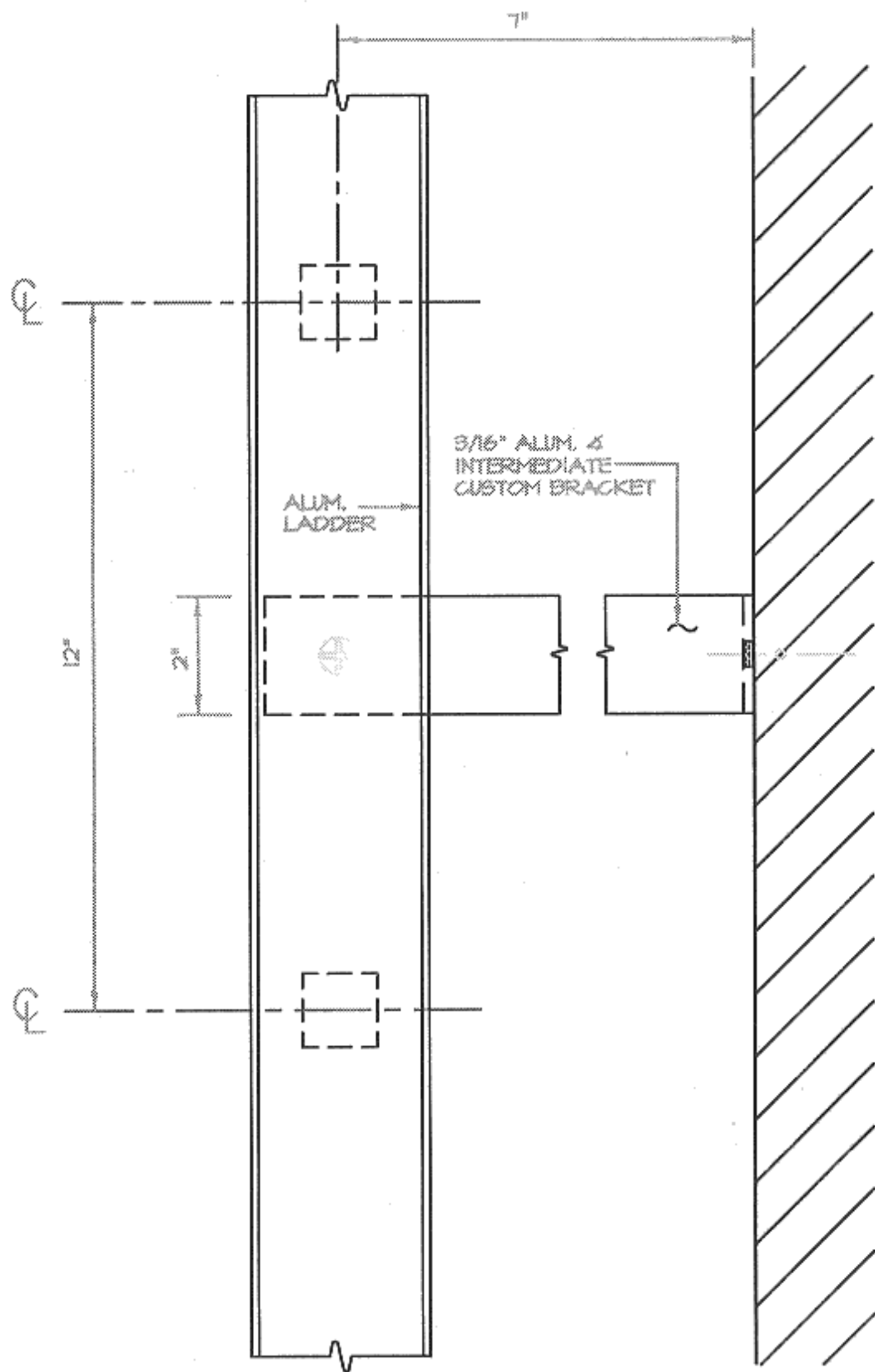
INTERMEDIATE BRACKET SCALE: 3"=1'-0"
